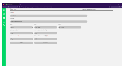
Editar Item
