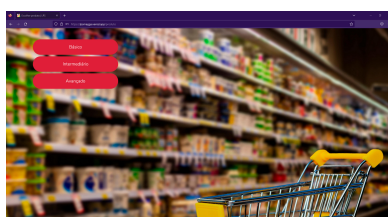
Escolher Produto
