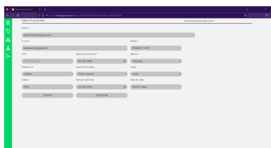
Editar Funcionário
