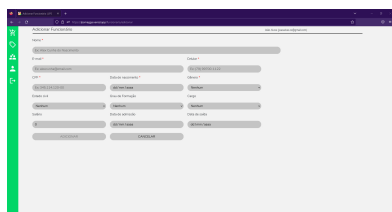
Adicionar Funcionário
