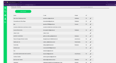
Manipular Cliente
