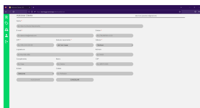
Adicionar Cliente
