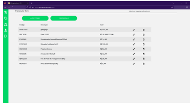
Manipular Item
