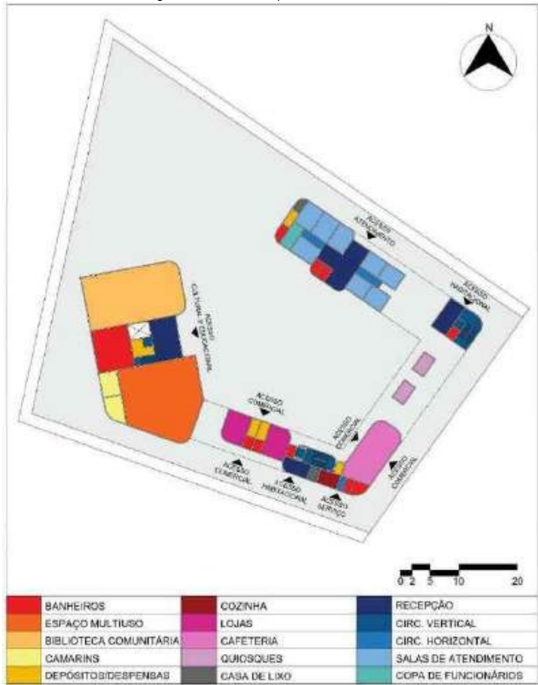
Figura 67 - Planta Esquemática do Térreo
