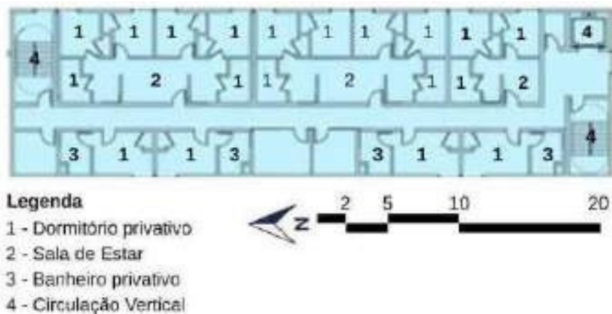
Figura 19 - Planta do 2º e 3º pavimentos do bloco de habitação temporária.
