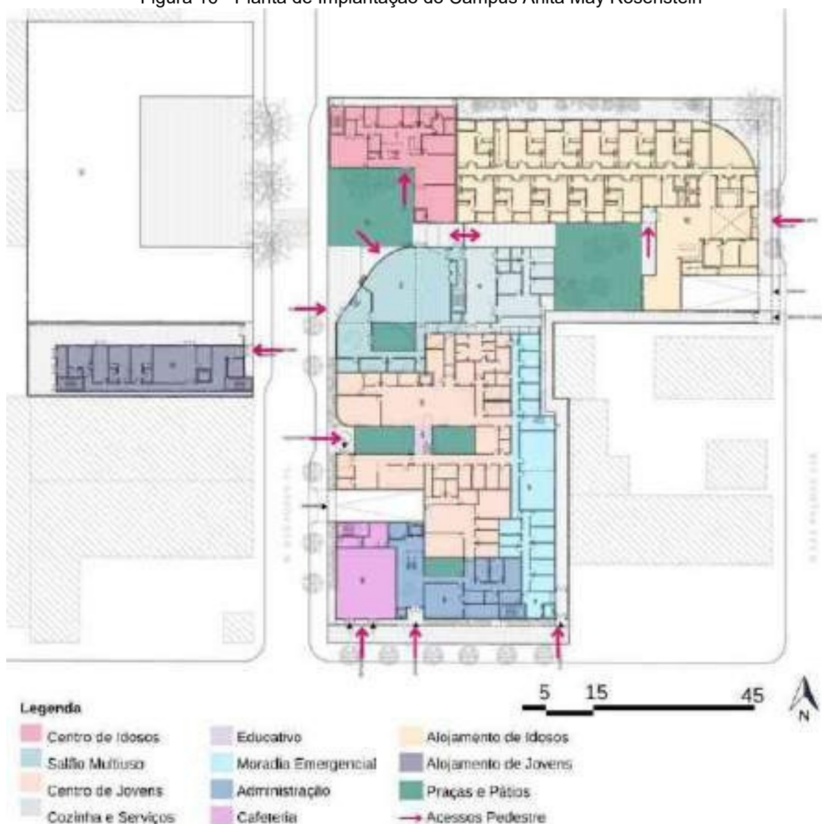
Figura 16 - Planta de Implantação do Campus Anita May Rosenstein
