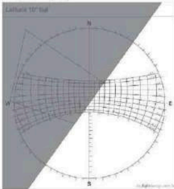
Figura 53 - Estudo de Incidência Solar através da Carta Solar 10° Sul
