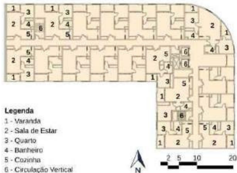
Figura 20 - Planta do 2º e 3º pavimento do alojamento de idosos.
