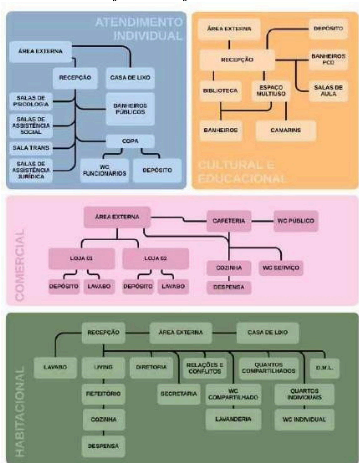
Figura 59 - Funcionograma de Ambientes
