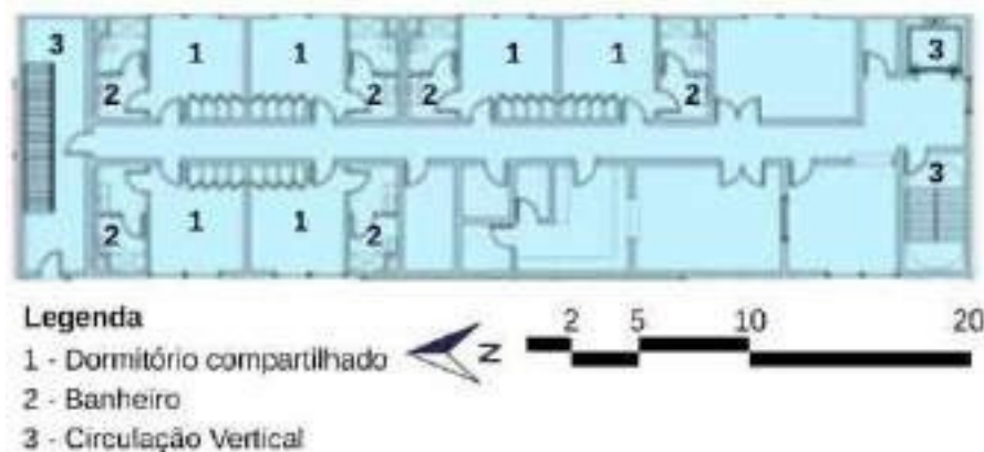
Figura 18 - Planta do 1º pavimento do bloco de habitação temporária
