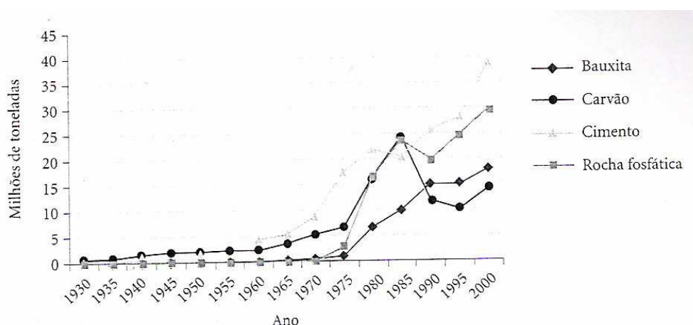
Figura 5.8 – Produção Mineral Brasileira – Bauxita, Carvão, Cimento e Rocha fosfática Fonte: SANCHEZ, L. E. A produção mineral brasileira: cinco séculos de impacto ambiental. In: RIBEIRO, C. W. (Org.). Patrimônio Ambiental Brasileiro . São Paulo: Edusp, 2003, p.135.
