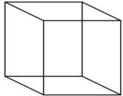
Figura 4.3: Hexaedro - 6 faces quadriláteras.
