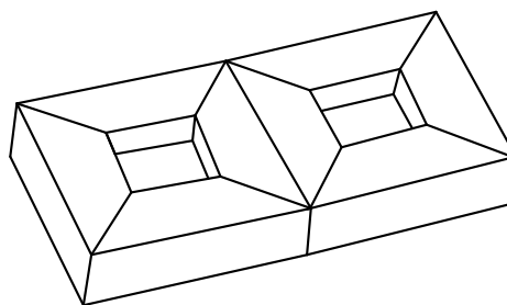
Figura 3.5: Poliedro não-convexo.
