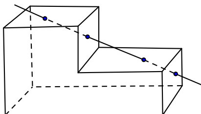
Figura 2.8: Poliedro não-convexo
