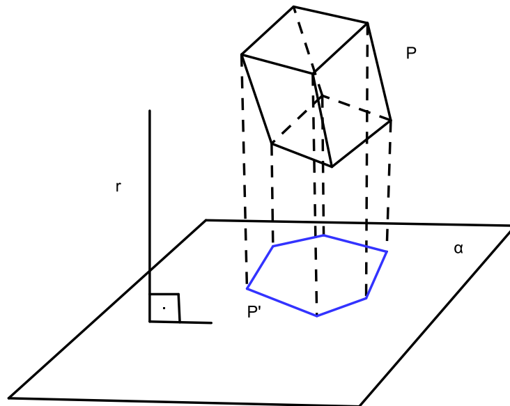
Figura 3.2: Projeção da sombra de um paralelepípedo, sendo que os raios de luz não incidem perpendicularmente a nenhuma face do paralelepípedo.
