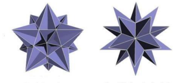
Figura 4.7: Grande Icosaedro e grande dodecaedro estrelado.
