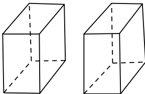
Figura 3.10: Objetos resultantes do corte.
