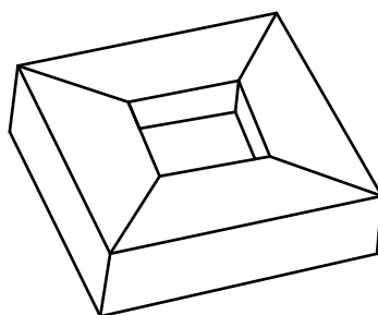
Figura 3.1: Poliedro não-convexo
