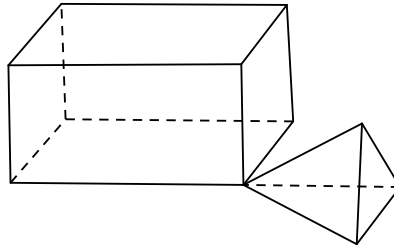
Figura 2.5: Objeto que não ilustra um poliedro
