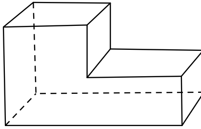
Figura 3.16: Poliedro não-convexo
