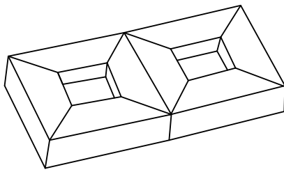
Figura 3.13: Poliedro não-convexo com gênero g = 2 .
