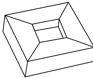
Figura 3.17: Poliedro não-convexo
