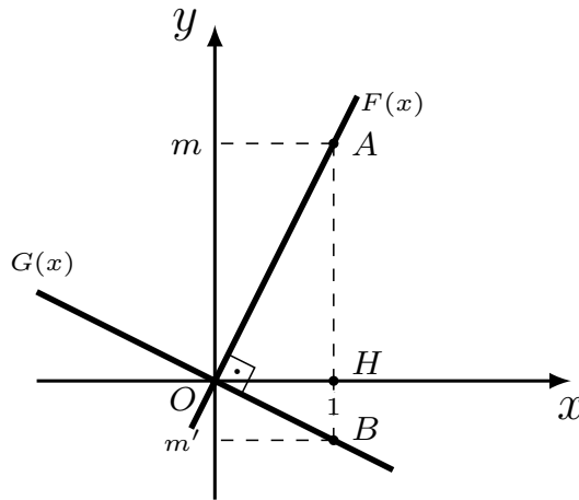
Figura 26 – Gráficos de F e G .
