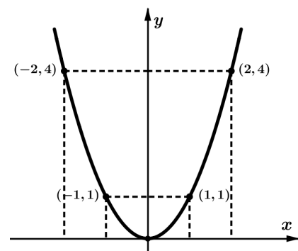
Figura 5 – Gráfico de f(x) = x^2 .
