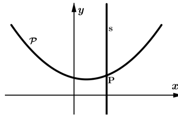
Figura 14 – A reta s não é tangente à parábola \mathcal{P} .
