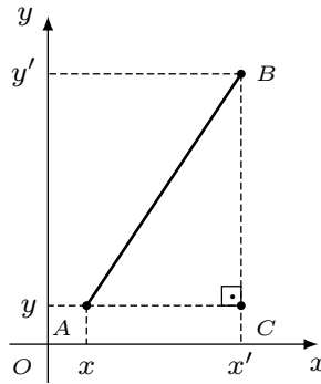
Figura 44 – Distância entre os pontos A e B .
