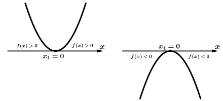
Figura 22 – Se \Delta = 0 , a \cdot f(x) \geq 0 .
