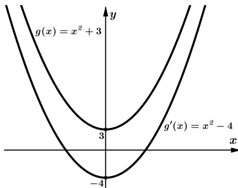
Figura 11 – Gráficos de g(x) = x^2 + 3 e g'(x) = x^2 - 4 .
