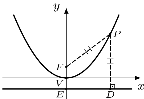
Figura 7 – Parábola de foco F e diretriz d = \overleftrightarrow{ED} .
