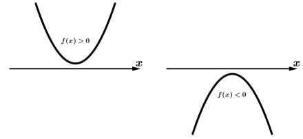
Figura 21 – Se \Delta < 0 , a \cdot f(x) > 0 .
