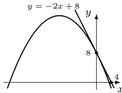
Figura 10 – Tangente ao gráfico de f(x) = -0,1x^2 - 2x + 8 .
