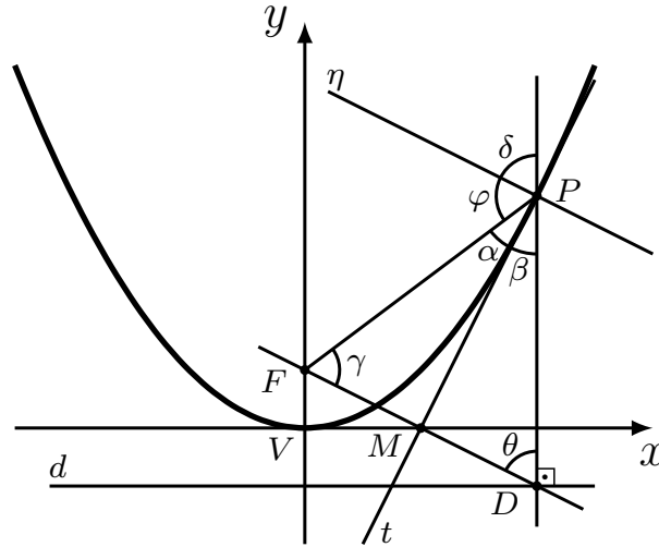
Figura 27 – A propriedade refletora da parábola.
