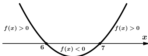
Figura 24 – Estudo de sinal do Exemplo 3.3.6.
