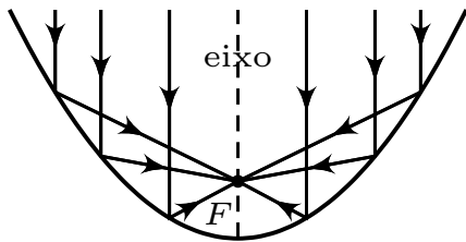
Figura 28 – Reflexão da luz.
