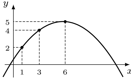
Figura 3 – Função quadrática definida pelos pontos (1, 2) , (3, 4) e (6, 5) .
