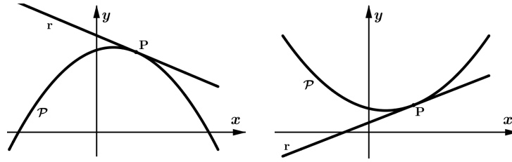
Figura 13 – Reta r tangente à parábola \mathcal{P} .
