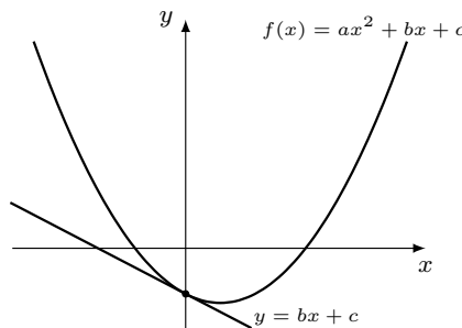
Figura 9 – Reta tangente no ponto (0, c) .
