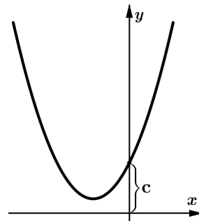
Figura 12 – y -interseção: (0, c) .
