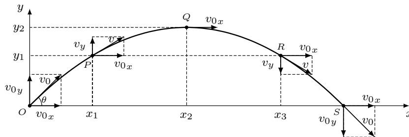
Figura 33 – Lançamento de um projétil.
