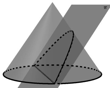
Figura 6 – Parábola: interseção de um cone e um plano paralelo a uma de suas geratrizes.
