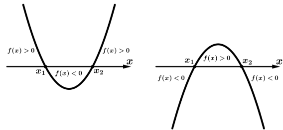
Figura 23 – Se \Delta > 0 , a \cdot f(x) \leq 0 sse x \in [x_1, x_2]
