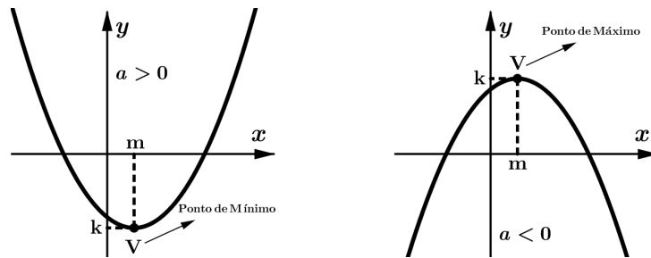
Figura 4 – Extremos da função quadrática.
