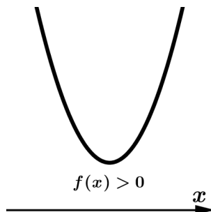
Figura 25 – f(x) tem o mesmo sinal de a quando \Delta < 0 .
