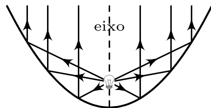
Figura 29 – Fonte luminosa no foco.
